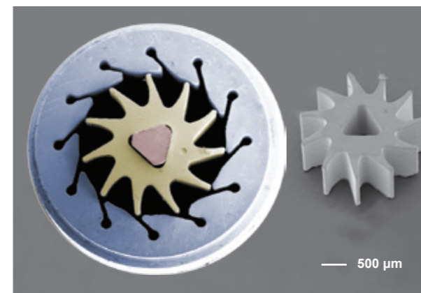
Mikroturbine (links) und Rotor der Mikroturbine aus Zirkonoxid (rechts)
