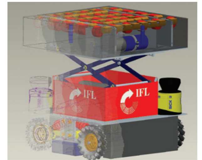
Abb. unten: Kleinskaliges Autonomes Redundantes IntraLogistik System Karlsruhe-Element mit Hub
