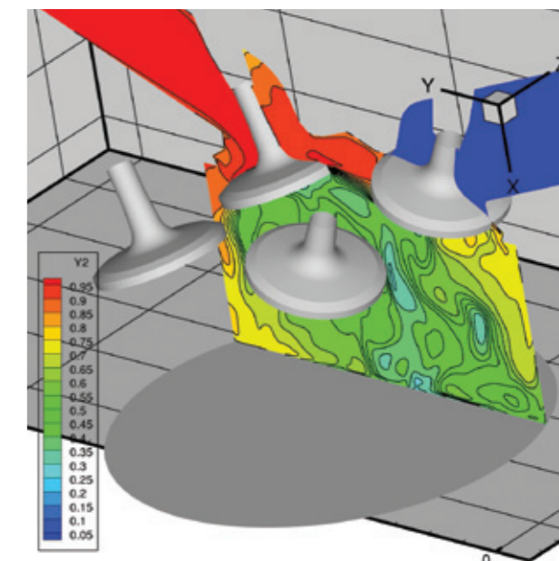
Einstromung des Benzin-Luftgemisches in den Zylinderraum eines Ottomotors
